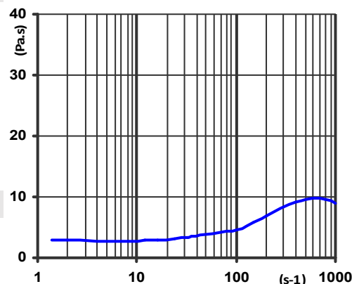
粘度曲线
