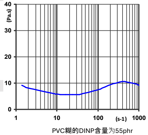
粘度曲线
