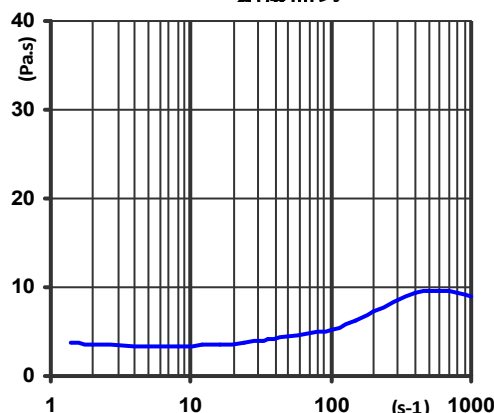
粘度曲线
